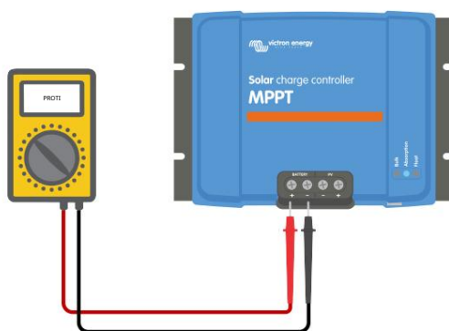
Měření napětí baterie na svorkách baterie ovladače
