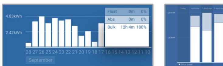
Systém tráví veškerý čas ve velkém s rozčleněním nabíjecích stupňů - Systém ve velkém a absorpce
